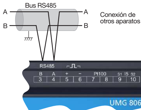
Fig. de ejemplo: Interfaz RS485 del UMG 806 (en medio de una topología de bus)
