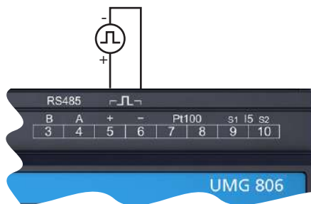
Fig.: Ejemplo de conexión: salida digital
