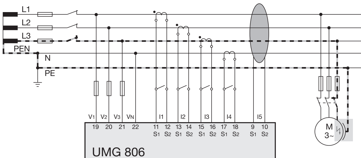
Fig. Ejemplo de conexión UMG 806 con monitorización de la corriente diferencial
