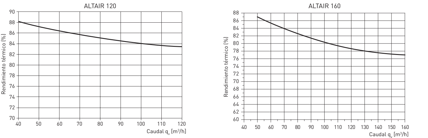
Rendimiento obtenido según UNE 13141-7 (Text 20°C y Tint 7°C).
