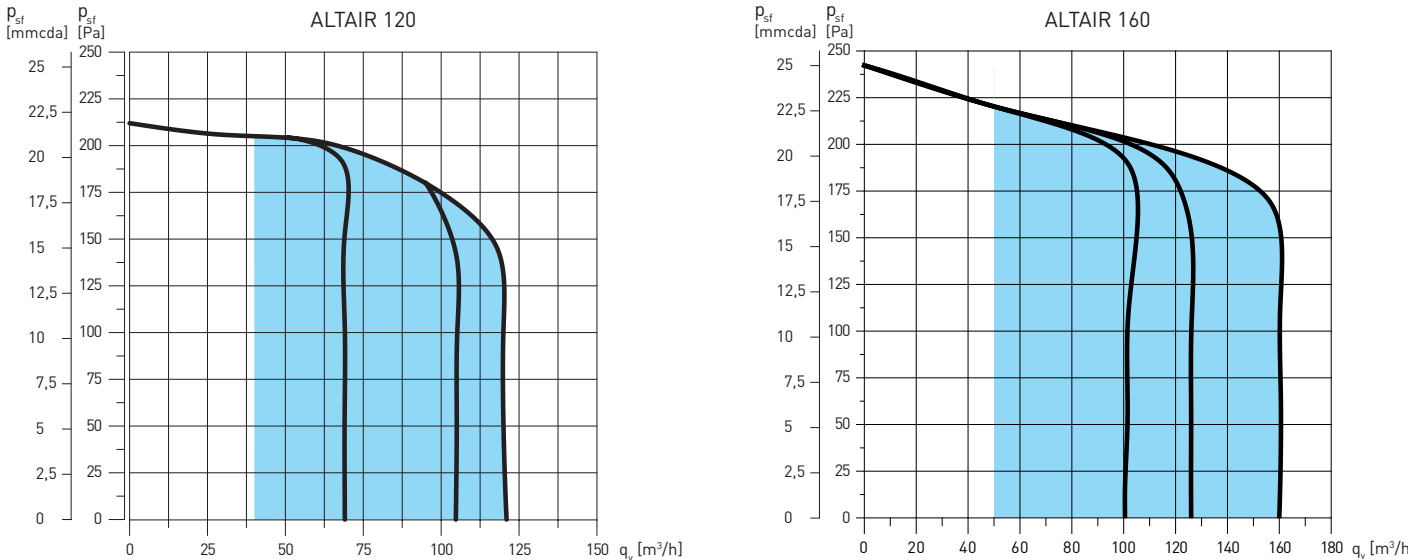
Curvas definidas considerando los filtros limpios.
